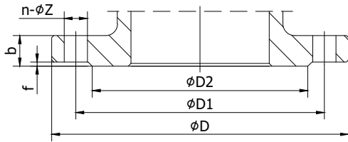
DIN 2543 PN16 Flanges
