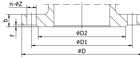
JIS B 2220 16K Flanges
