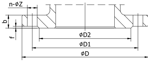
JIS B 2220 10K Flanges
