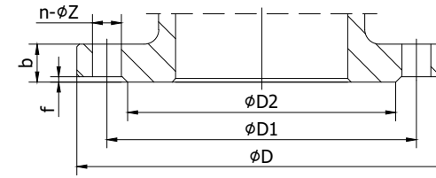
JIS B 2220 20K Flanges
